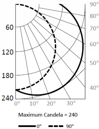
LEDUC-E24 (865 Lumens)
